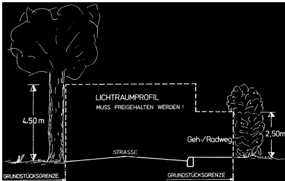
Schematische Darstellung mit den erforderlichen Maßen im öffentlichen Verkehrsraum
